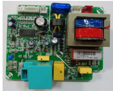
برد کنترل پارلار B3315if 20009209
